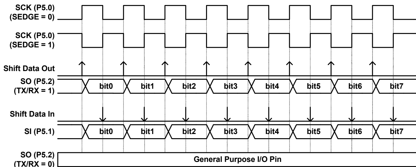
SIO 数据传输时序图
