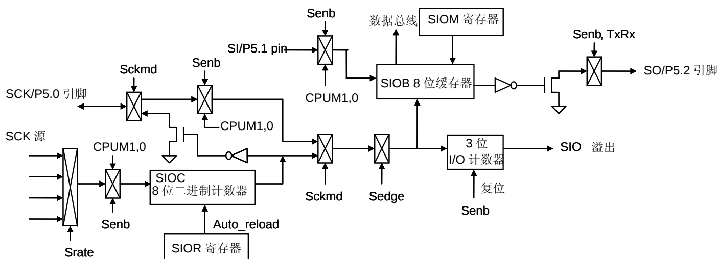
SIO 接口电路图
