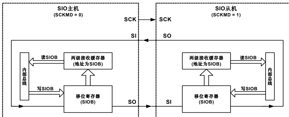
SIO 数据传送示意图
