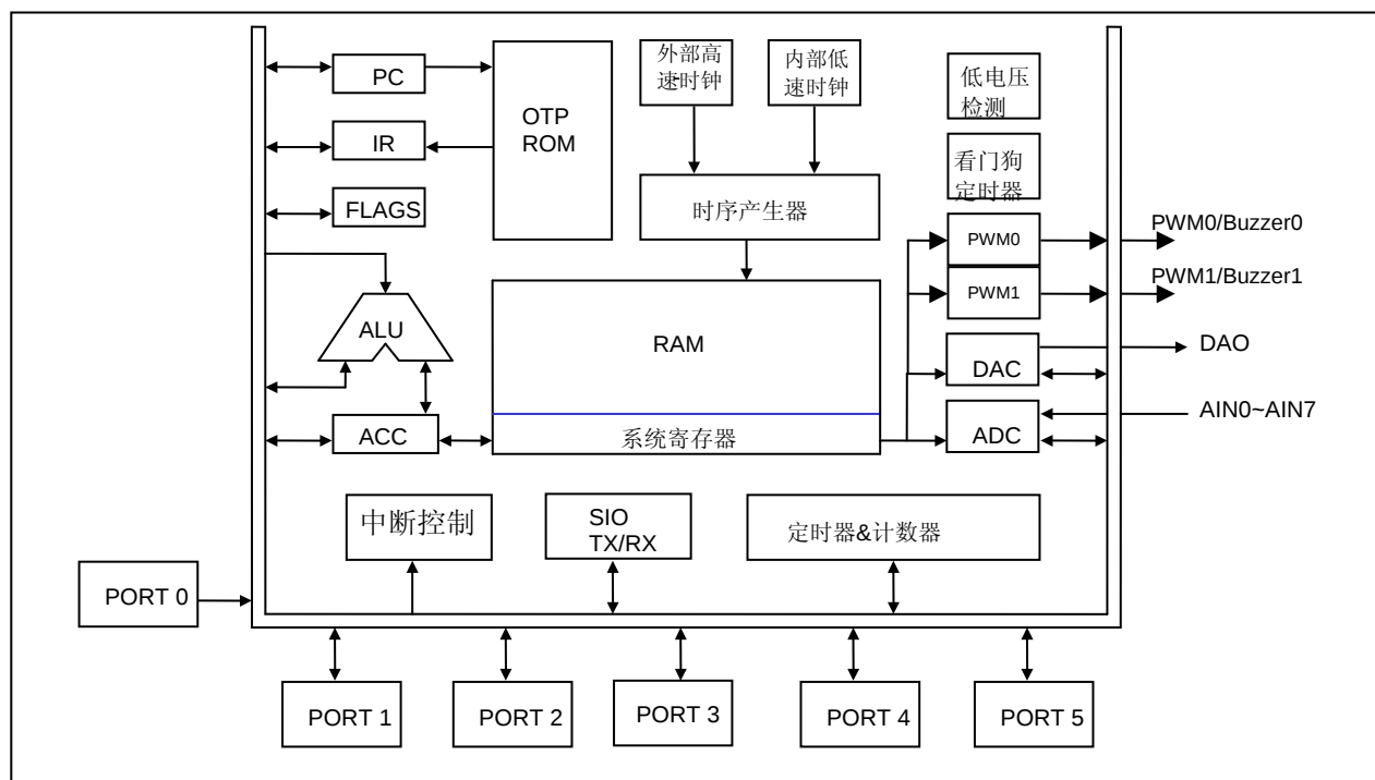
系统框图
